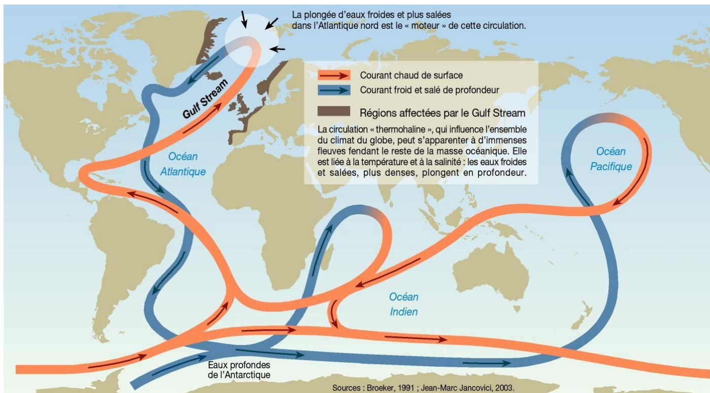
Schéma montrant le trajet des courants marins
